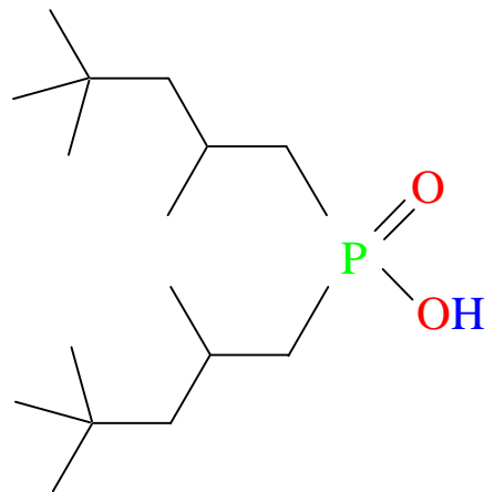
H[TMPeP] (LN3)
